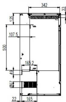
Prerez/Section A-A
