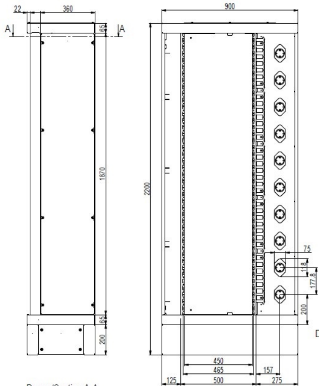
Prerez/Section A-A
