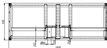
Prerez/Section A-A
